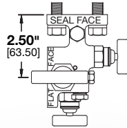
M3-875 (Patented)
