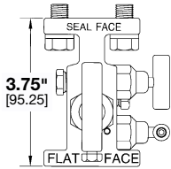
M3-775
